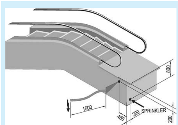
FIG. 13 SPRINKLER PIPING
